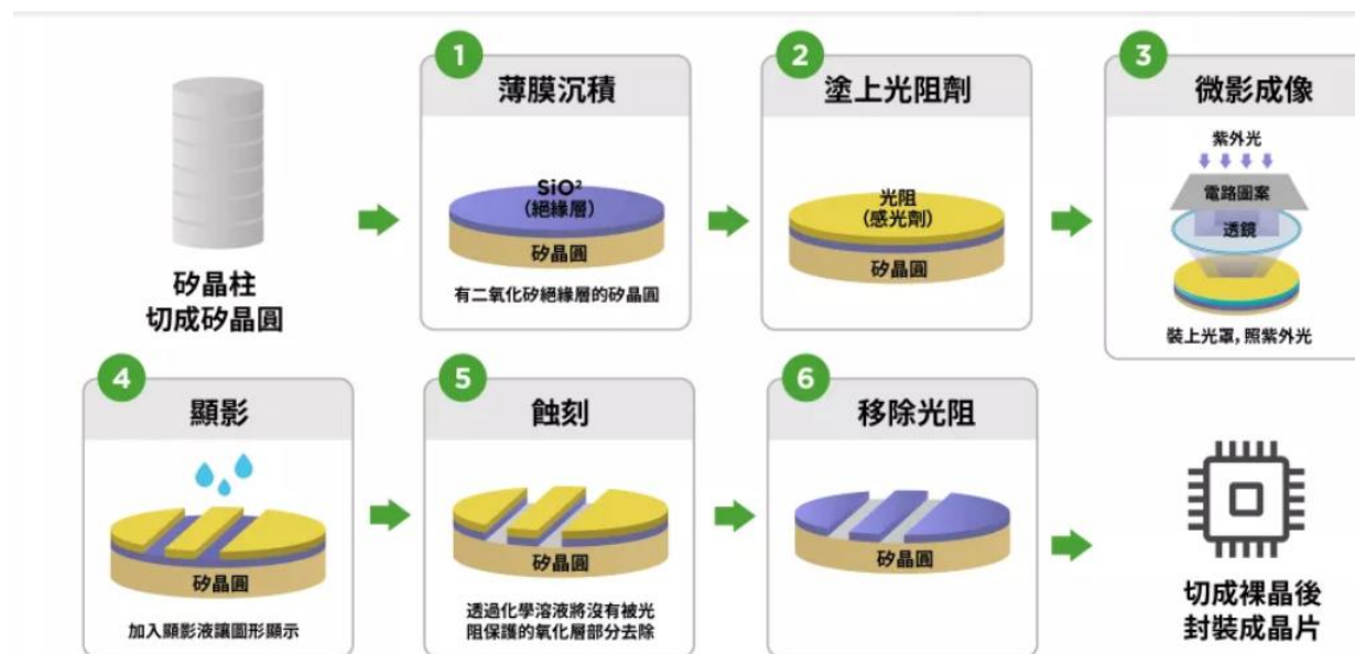
半導體製程流程圖
